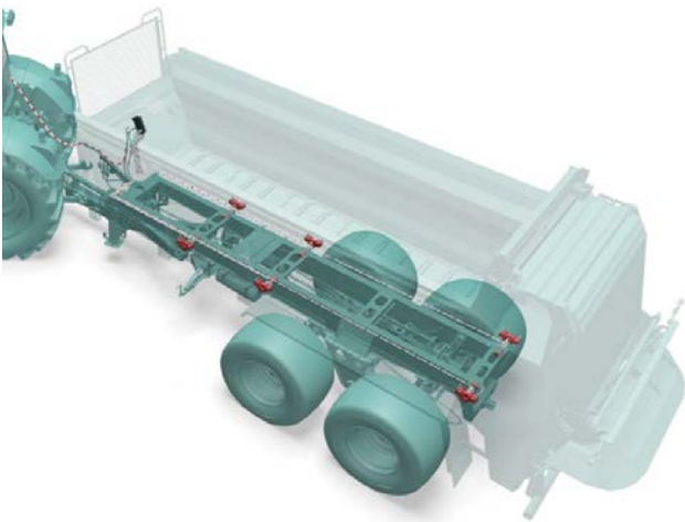
Spridarens flak ligger på vågceller som hela tiden väger lasten och justerar spridningsmängden konstant för att nå önskad spridningsmängd.
